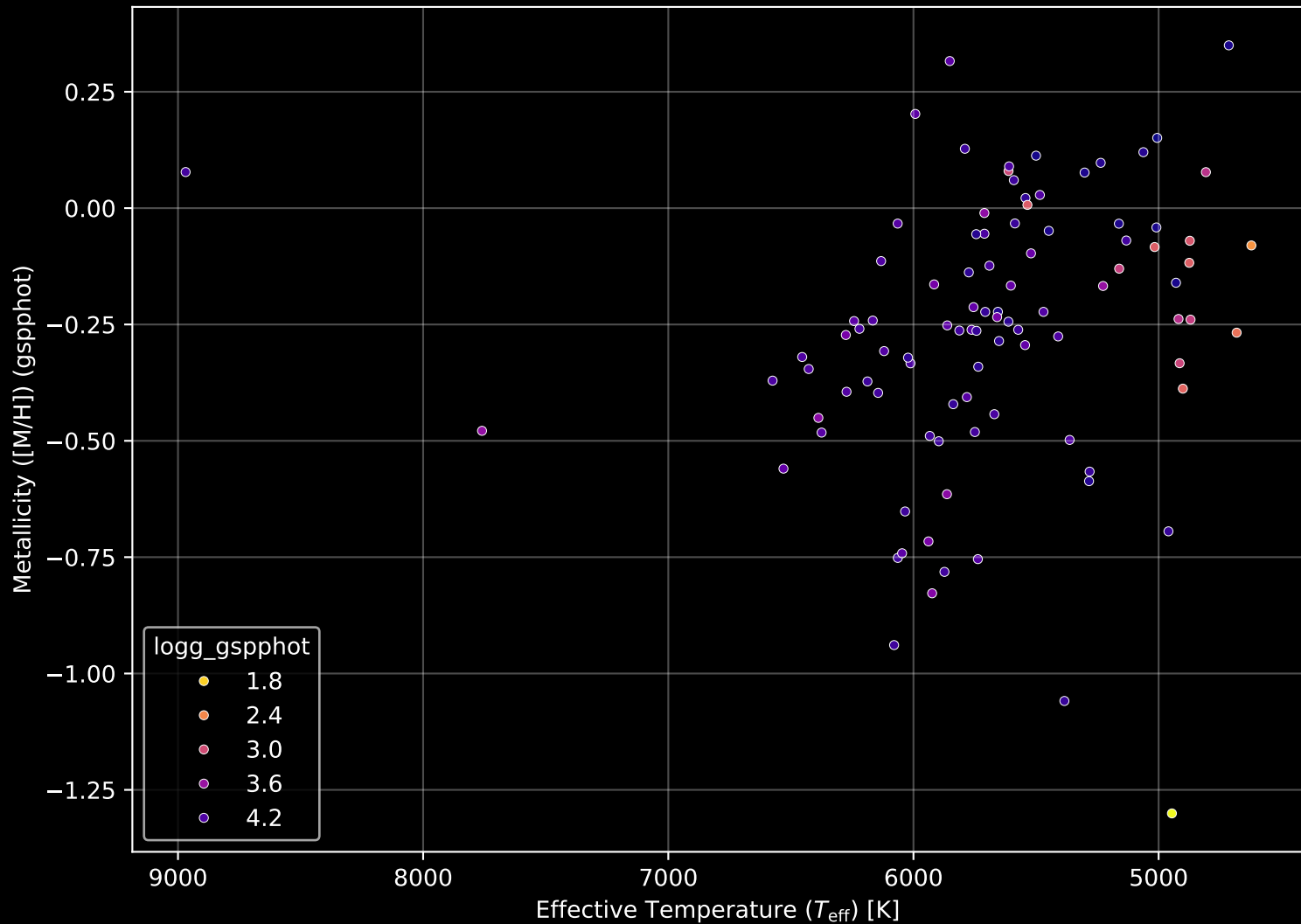
GALAH DR4 Field: [6684] Stellar Population Parameters (n= 97)
