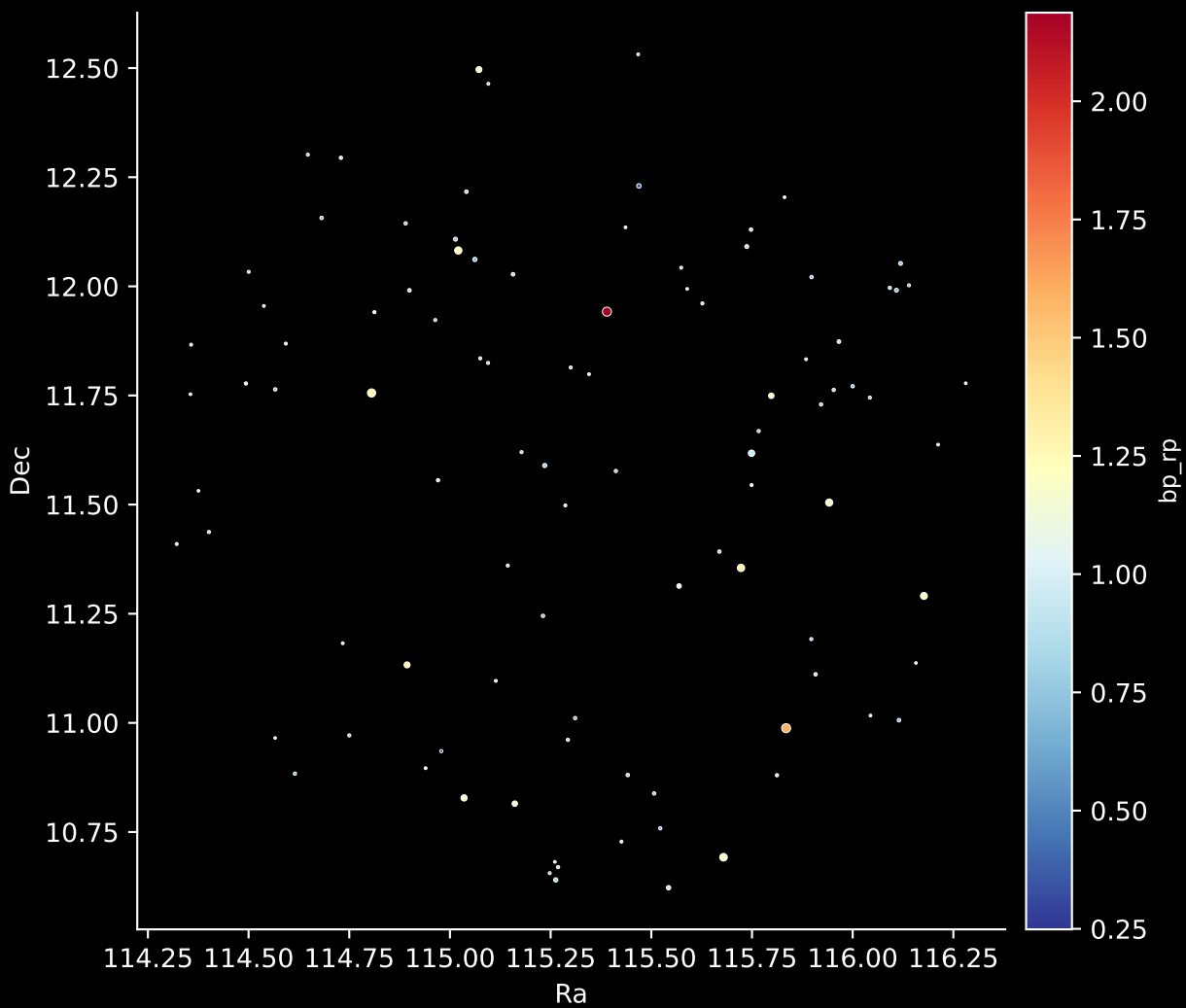
GALAH DR4 Field: [6684] Stars: 97
